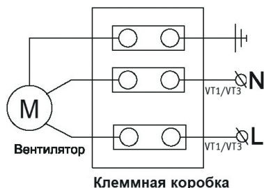
Клеммная коробка
