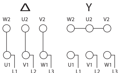
Рисунок А.1.2 - Схема подключения двигателя с соединением фаз обмотки «Δ/У» (шесть выводных концов)
