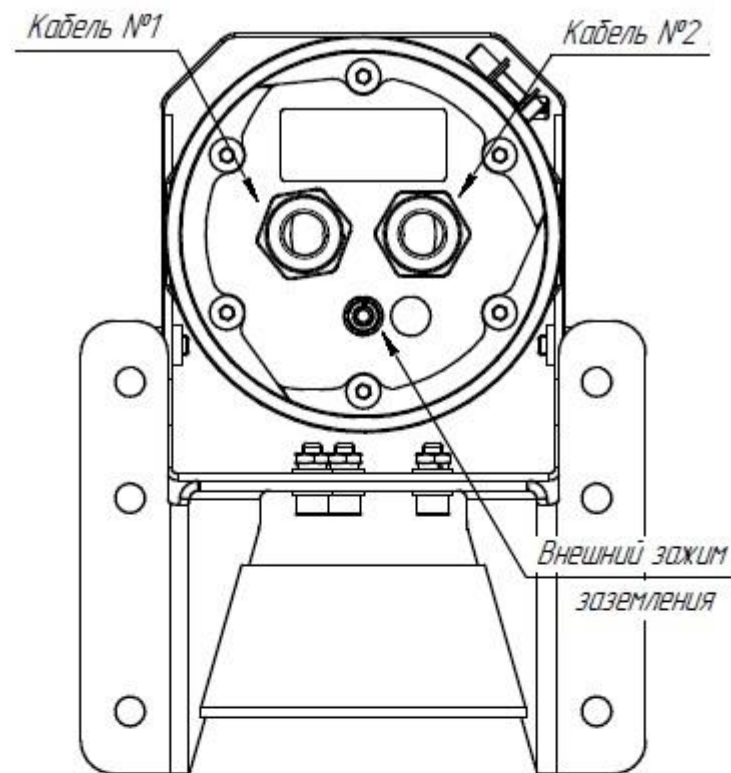
Кабель №1 КСКПП-ВПнз(А)-НФ 6х2х0.2; длина 1 м.
