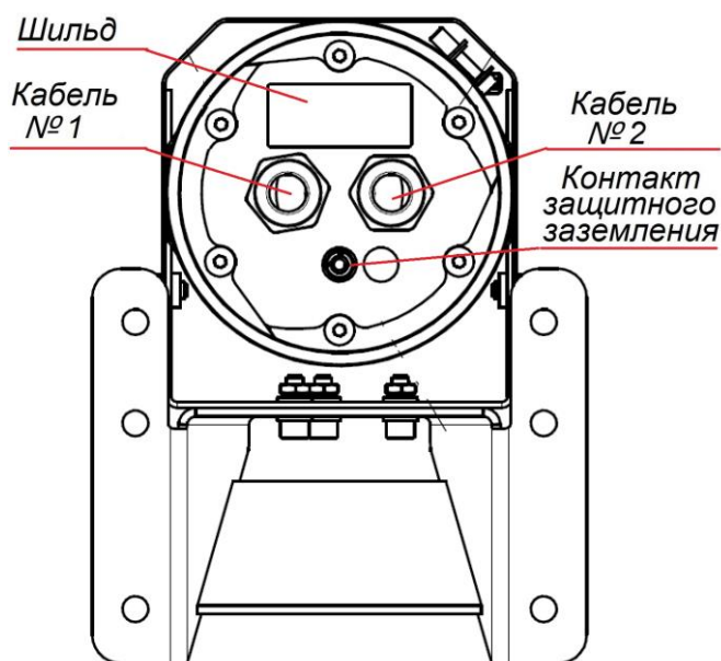
Рис.5.3.1 Вид термокожуха BCM-250Ex сзади
