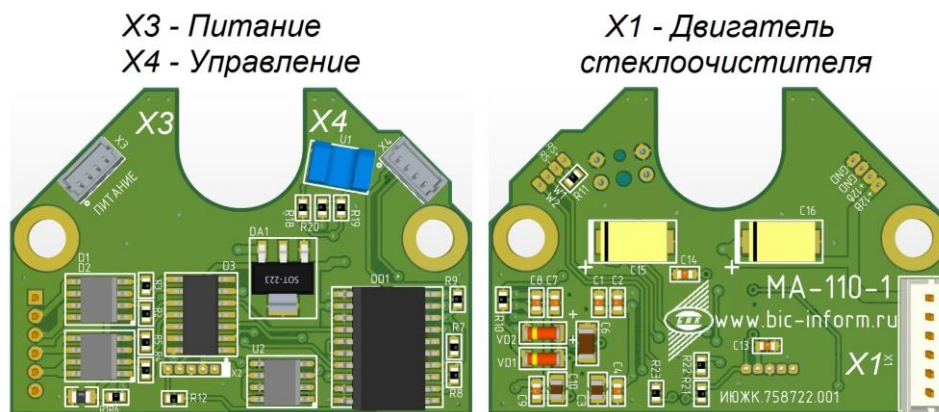
Рис.5.1.3 Внешний вид платы контроллера дворника МА-110 и расположение элементов коммутации
