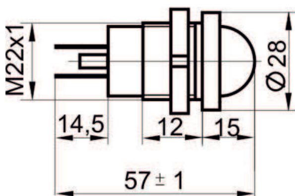
Габаритные размеры
