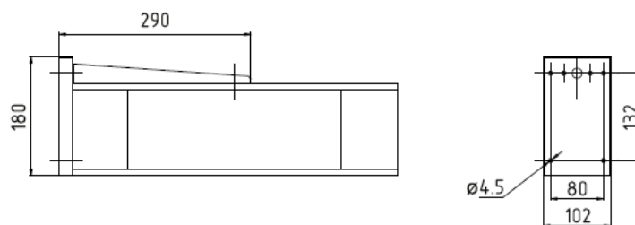
Кронштейн BS-K-2
