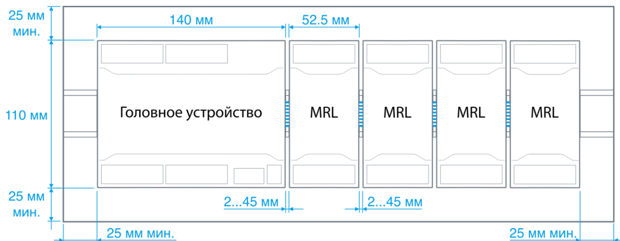
Рис. 8 - Пример компоновки
