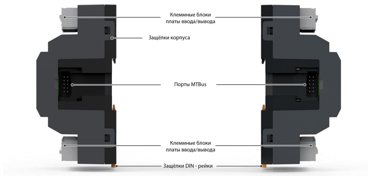
Рис. 4 – Модуль ввода/вывода, виды сбоку
