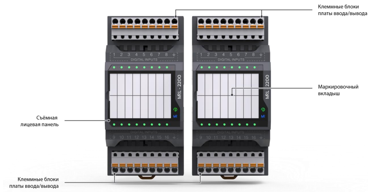
Рис. 3 – Модуль ввода/вывода, вид спереди
