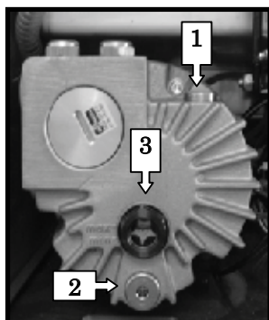
Вид сзади JUMBO PLUS (задняя панель снята)
