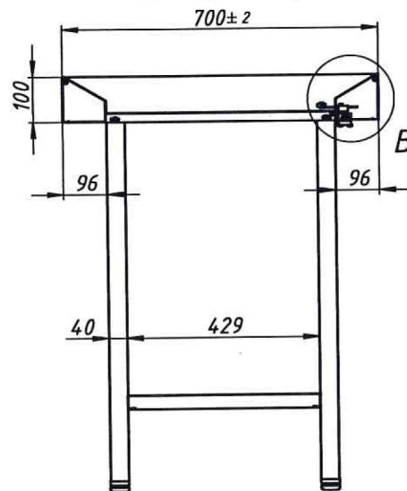
A-A (1:10)
