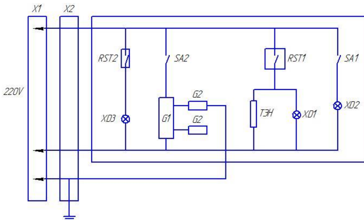
Схема электрическая принципиальная для духовки
