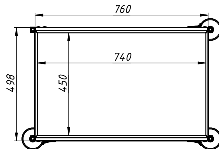
A-A ( 1 : 10 )
