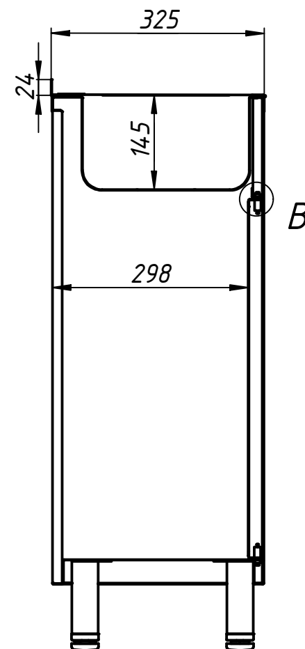
A-A (1:8)
