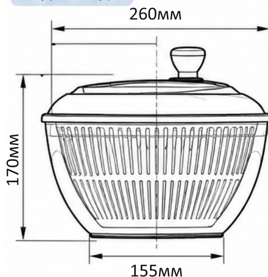
ВИД СПЕРЕДИ
