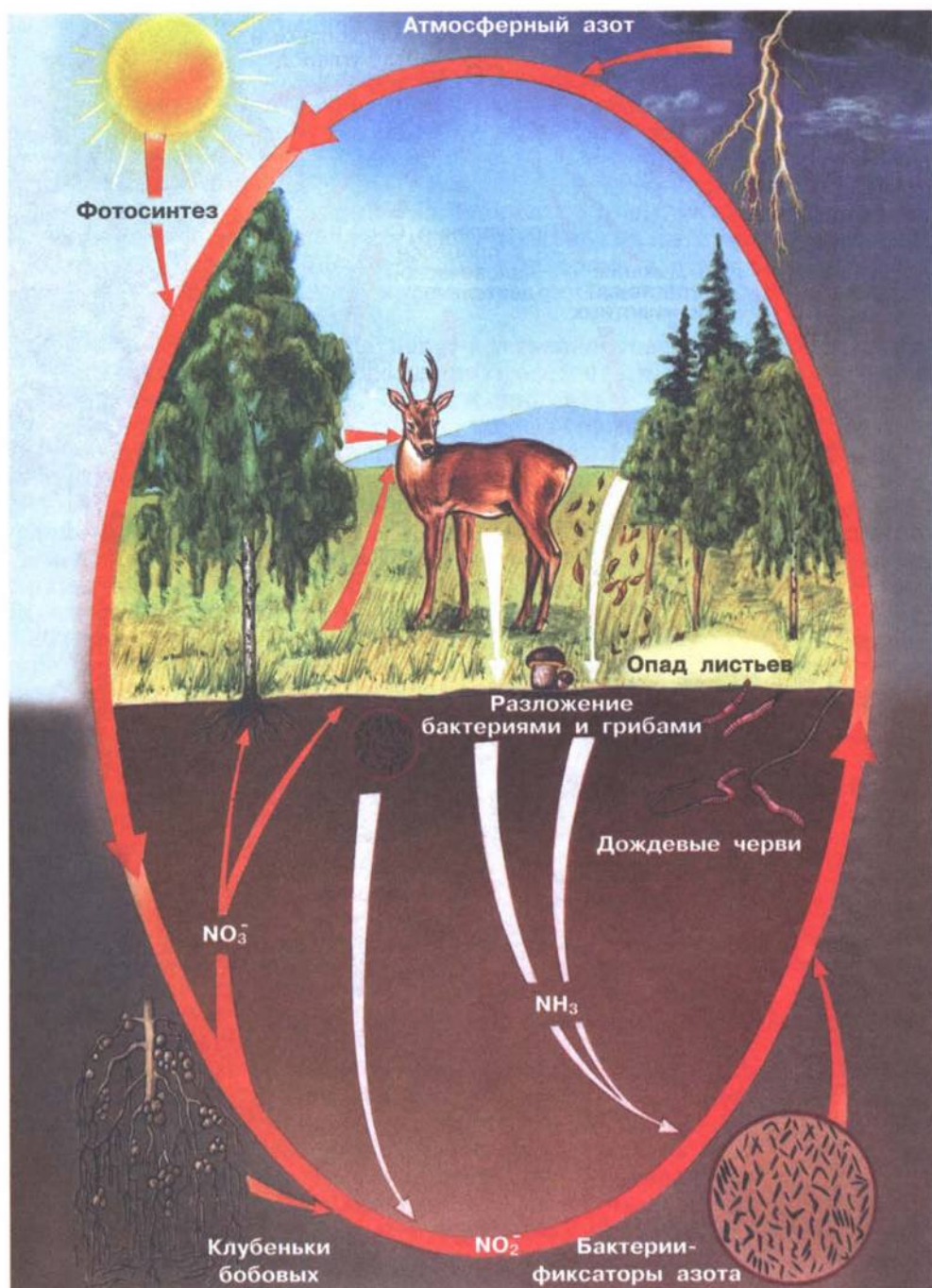
Рис. 108. Круговорот азота
