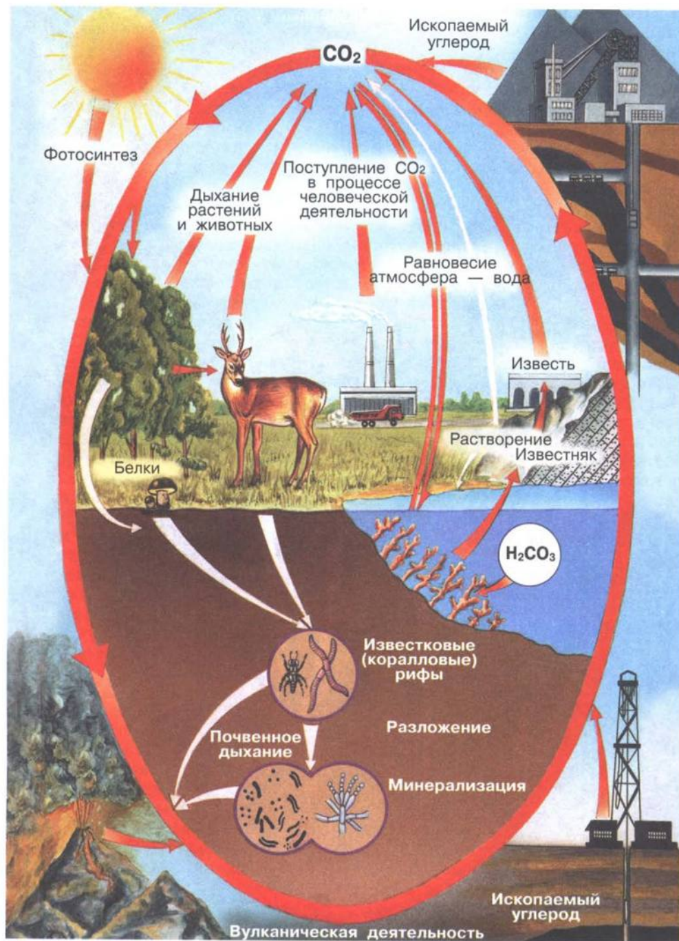
Рис. 107. Круговорот углерода
