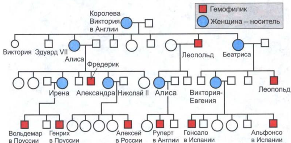
Рис. 46. Наследование гемофилии
