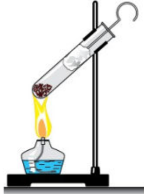
Рис. 89. Получение белого фосфора из красного
