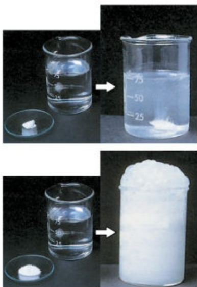
Рис. 103. Зависимость скорости химической реакции от площади соприкосновения реагирующих веществ
