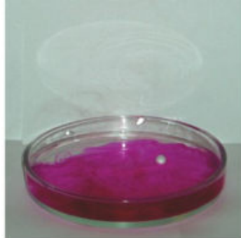
Рис. 96. Взаимодействие натрия с водой, в которую добавлен фенолфталеин
