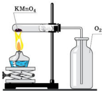
Рис. 59. Получение кислорода в лаборатории разложением перманганата калия и соби́рание его методом вытеснения воздуха
