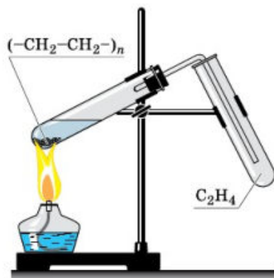
Рис. 150. Прибор для получения этилена деполимеризацией полиэтилена
