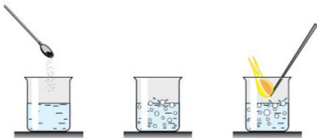
Рис. 105. Разложение пероксида водорода с использованием оксида марганца (IV)
