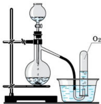
Рис. 60. Получение кислорода в лаборатории разложением пероксида водорода и соби́рание его методом вытеснения воды
