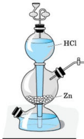
Рис. 53. Аппарат Киппа
