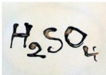
Рис. 129. Обугливание бумаги концентрированной серной кислотой
