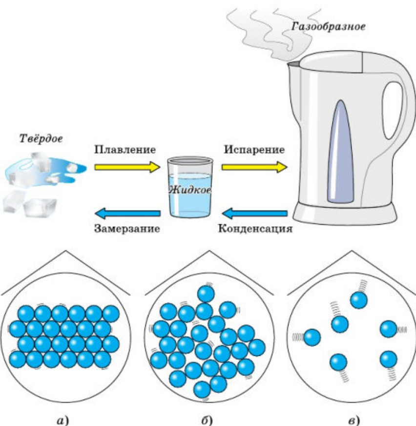
Рис. 50. Агрегатные состояния воды: а — твёрдое; б — жидкое; в — газообразное
