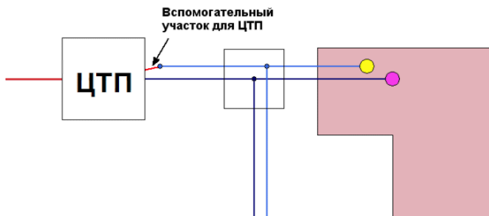
Рисунок 5. Подключение трубопровода ГВС Потребитель
