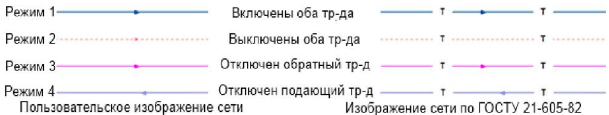
Рисунок 2. Изображение нескольких состояний участков, задаваемых разными режимами
