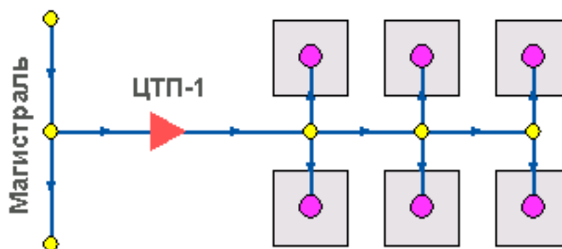
Рисунок 4. Изображение ЦТП
