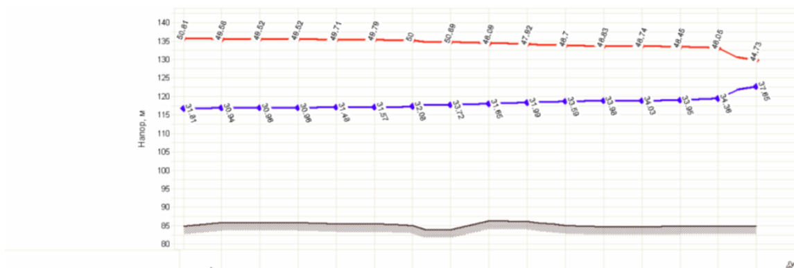
Рисунок 24. Пример пьезометрического графика
