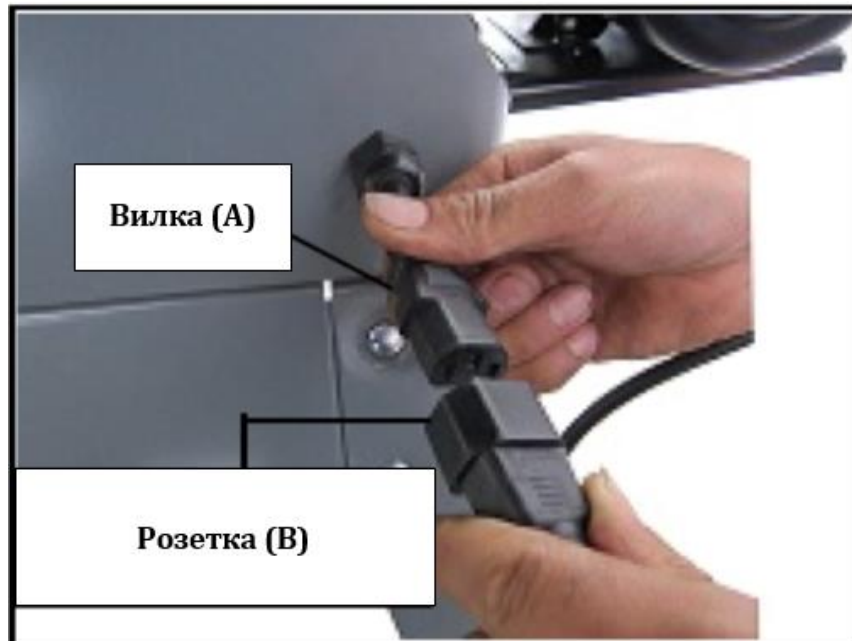
Рис. 31. Соединение вилка-розетка
