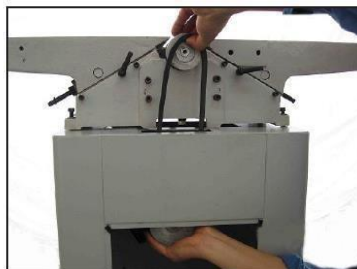
Рис. 6. Надевание клинового ремня
