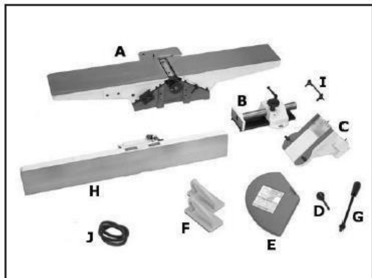
Рис. 1. Комплект поставки ящика 1
