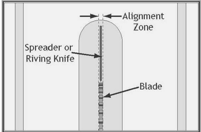
Рисунок 110. Зона выравнивания раскливающего ножа.
