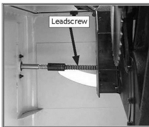
Рисунок 98. Ходовой винт.
