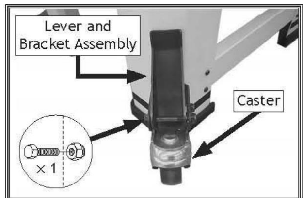
Рисунок 13. Ролик, установленный на передней правой ноге
