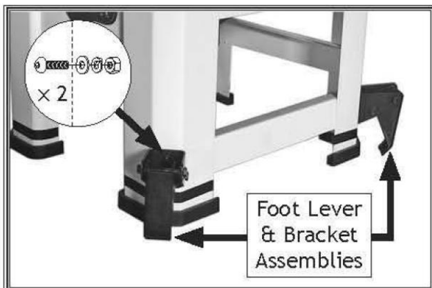
Рисунок 12. Установленные рычажные узлы.
