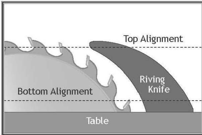
Рисунок 109. Пример проверки параллельности раскливающего ножа относительно пильного диска.
