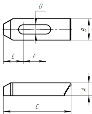
Прижим плоский
