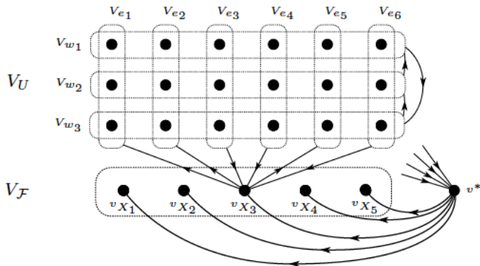
Рис. : Параметризованное сведение от задачи о покрытии множествами к задаче о доминирующем множестве в графах турнирах
