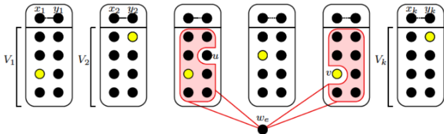
Рис. : Параметризованное сведение разноцветного независимого множества к доминирующему множеству
