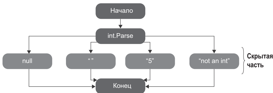
Рис. 1.6. Скрытые пути во внешних библиотеках. Метрики покрытия не видят, сколько существует таких путей и сколько из них будет отработано вашими тестами
