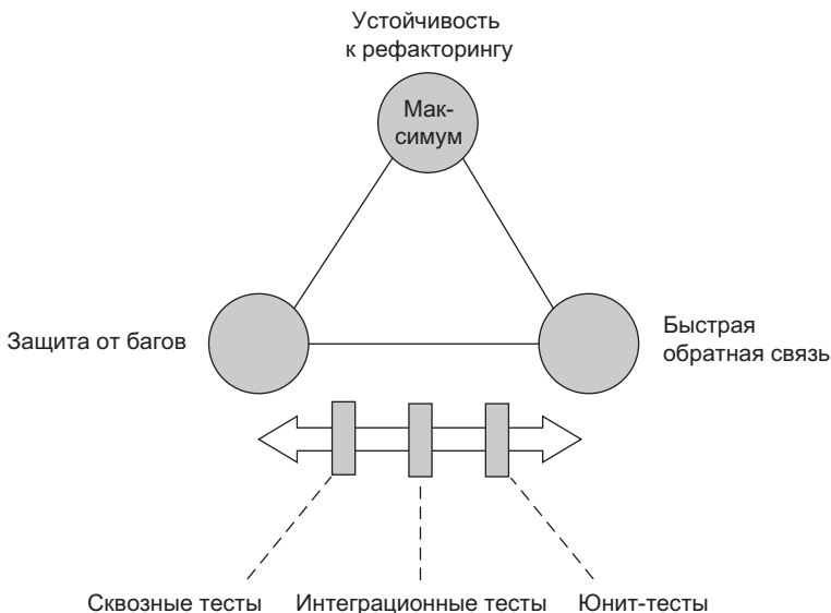
Рис. 4.12. Разные типы тестов в пирамиде принимают разные решения относительно быстрой обратной связи и защиты от багов. Сквозные тесты отдают предпочтение защите от багов, юнит-тесты — быстрой обратной связи. Интеграционные тесты находятся посередине
