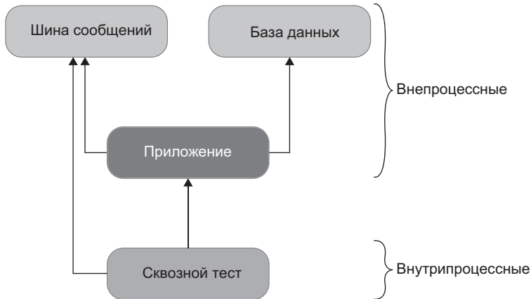
Рис. 8.7. Сквозные тесты эмулируют внешнего клиента и, как следствие, проверяют развернутую версию приложения вместе со всеми внепроцессными зависимостями, включающимися в сферу тестирования. Сквозные тесты не должны проверять управляемые зависимости (например, базы данных) напрямую — только косвенно, через приложение
