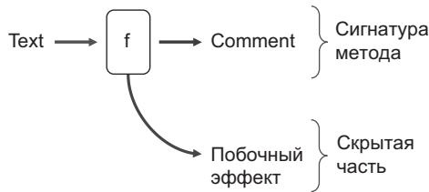
Рис. 6.8. Метод AddComment (представленный как f ) получает входное значение Text и возвращает значение Comment. Оба значения представлены в сигнатуре метода. Побочным эффектом является дополнительный скрытый результат
