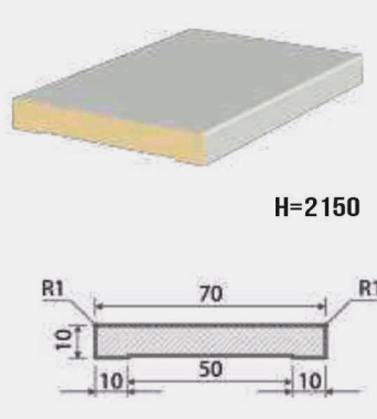
НАЛИЧНИК ПРЯМОУГОЛЬНЫЙ
