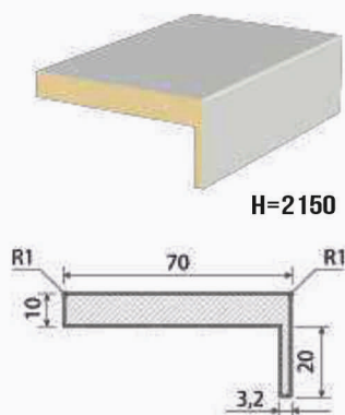
НАЛИЧНИК ТЕЛЕСКОПИЧЕСКИЙ
