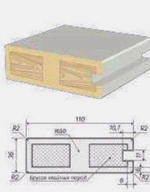
СТОЕВАЯ ЦАРГА
