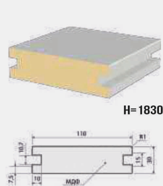
ПОПЕРЕЧНАЯ ПЛАНКА
