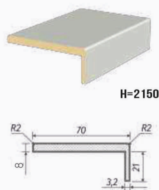
НАЛИЧНИК ТЕЛЕСКОПИЧЕСКИЙ
