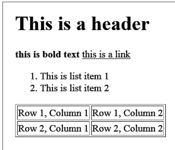
Рис. 12.1. Визуализированная HTML-страница
