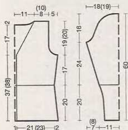
Схема к модели 5
