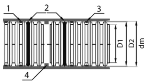
Монтаж соединительной муфты: 1, 3 – выступ, 2 – резиновое уплотнительное кольцо, 4 – ограничительный выступ муфты
