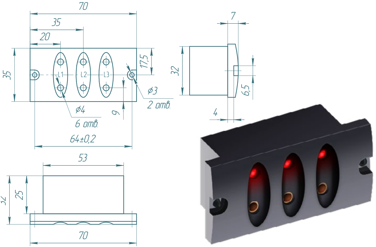
Габаритно-присоединительные размеры
