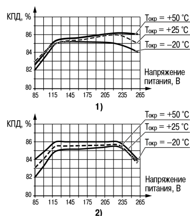
Рисунок 7 - График зависимости КПД от напряжения питания и температуры окружающей среды: (1) БП60А-12, (2) БП60А-24
