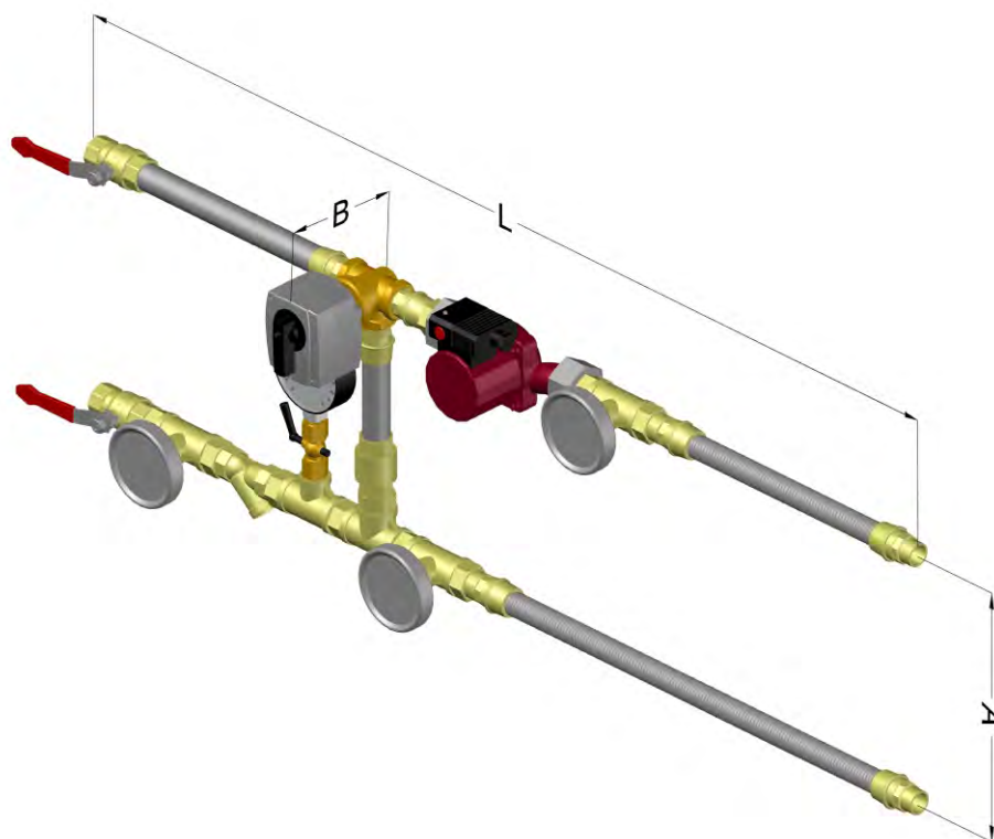
Узлы регулирования воздушонагревателей
