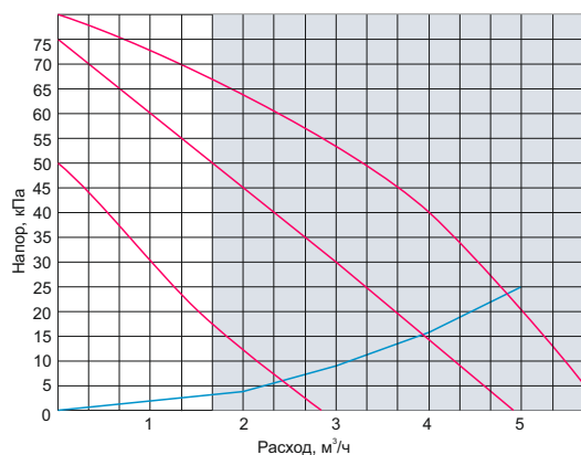
OD-25.0-40-120-P3-GL
