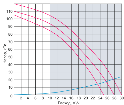
OD-60.0-65-120-P3-GL
