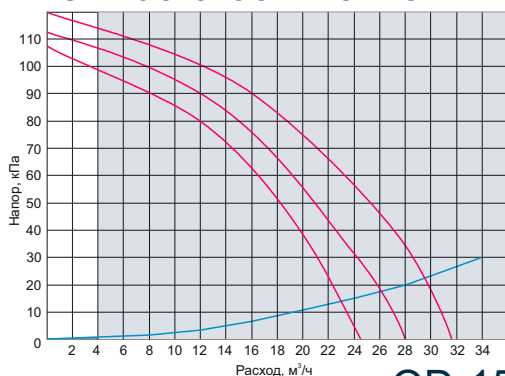
OD-60.0-65-120-P3-WL
