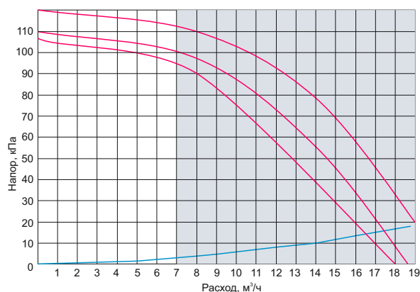
OD-90.0-80-120-P3-GL
