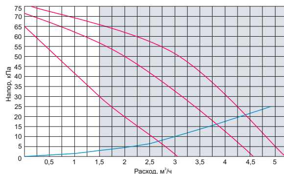
OD-16.0-32-120-P1-WL
