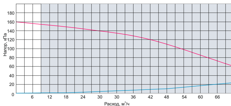
OD-150.0-100-160-P3-GL
