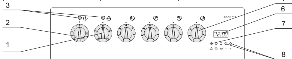
рис. 6. Панель плиты с электромеханическим таймером
