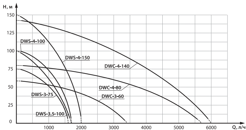
Рис. 2. График зависимости производительности от высоты подъема воды скважинных насосов Denzel: 97250, 97251, 97252, 97254, 97255, 97256, 97258.
