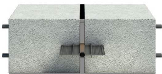
Рисунок 5.7 – Внутренняя гидрошпонка
