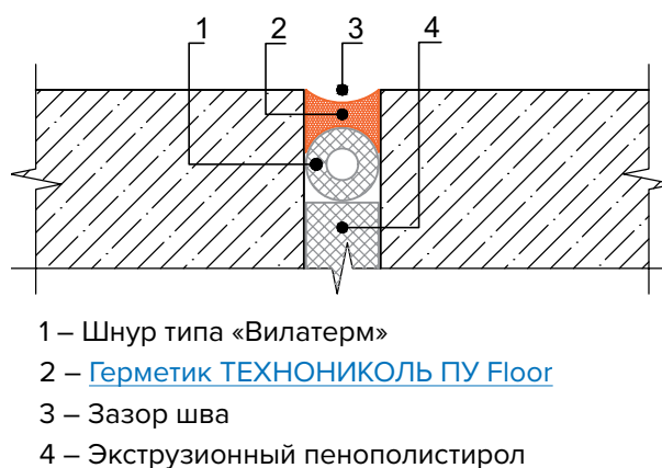
Рисунок 5.12 – Применение шнура из вспененного полиэтилена типа «Вилатерм»
