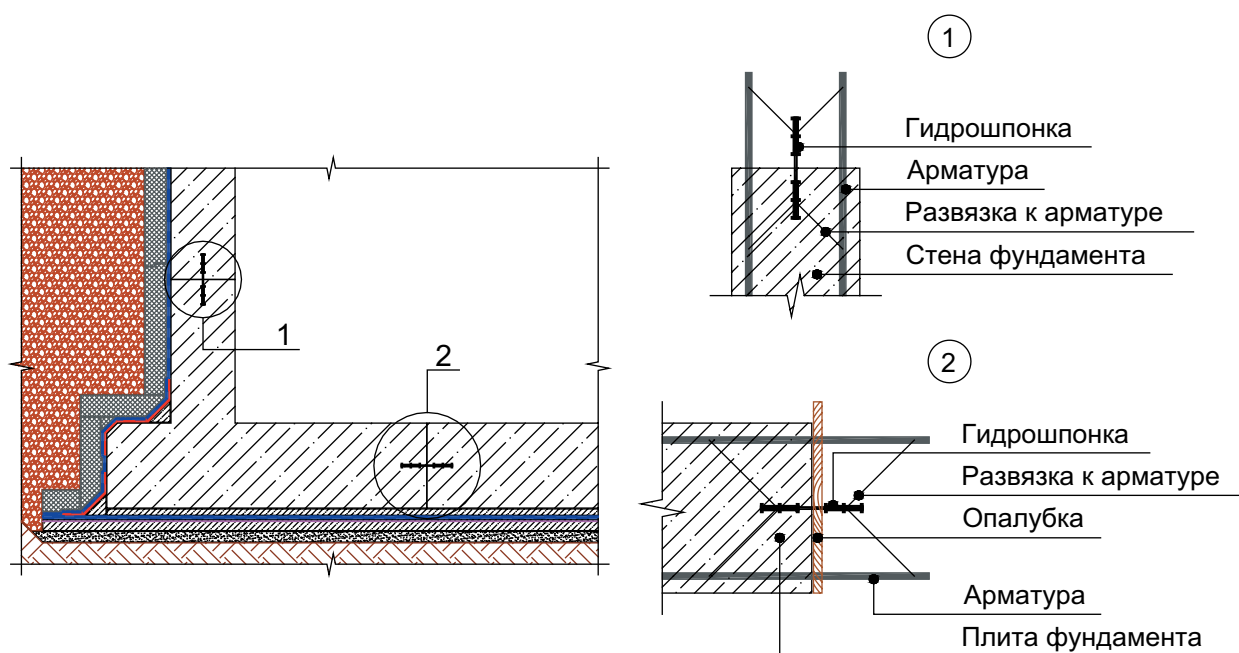
Рисунок 5.3 – Монтаж внутренней гидрошпонки для технологических швов
