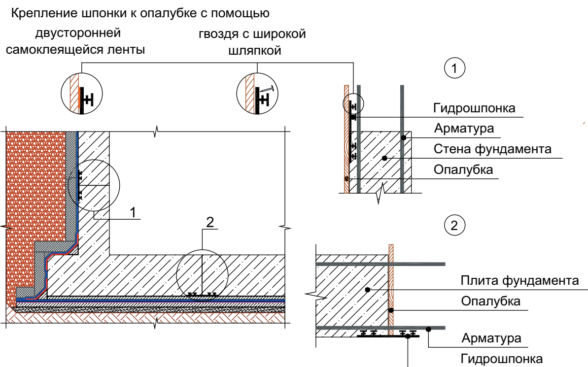
Рисунок 5.4 – Монтаж внешней гидрошпонки для технологических швов
