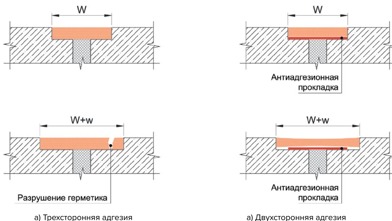
Рисунок 5.11 – Применение антиадгезионной прокладки в конструкциях Т-образного деформационного шва
