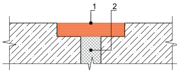
Рисунок 5.9 – Характеристики для определения коэффициента формы шва (K)
