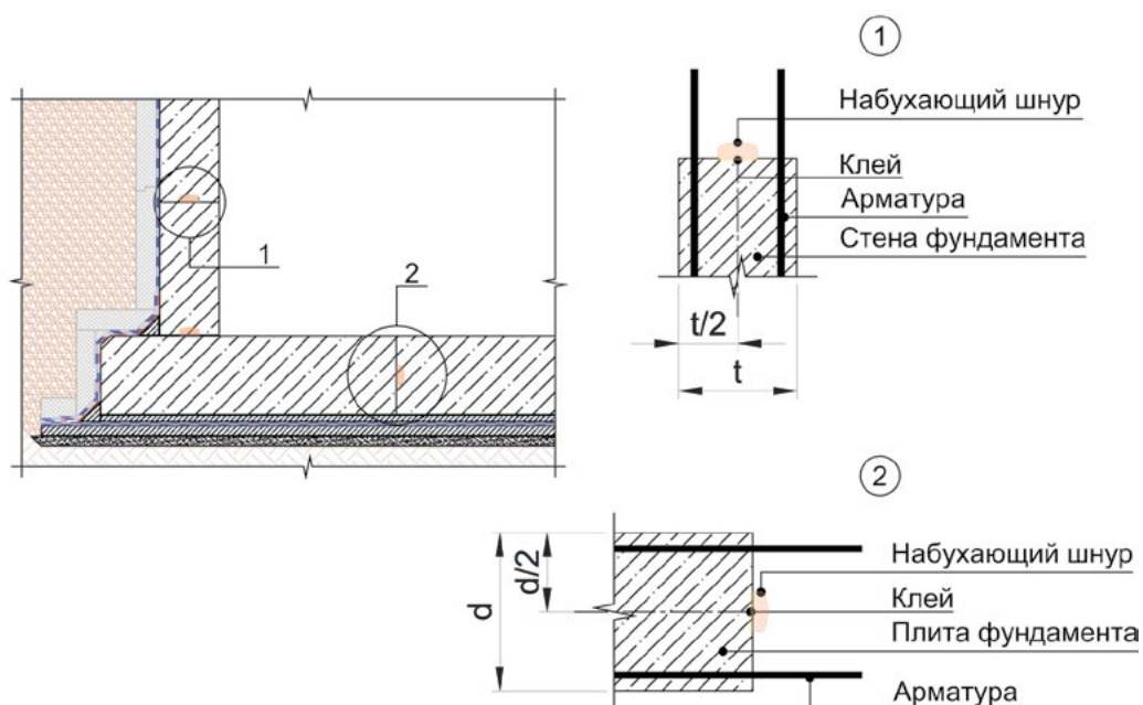
Рисунок 5.5 – Монтаж набухающих полимерных профилей для технологических швов
