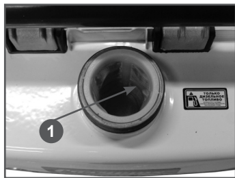
Рис. 8 Максимальный уровень топлива в топливном баке
