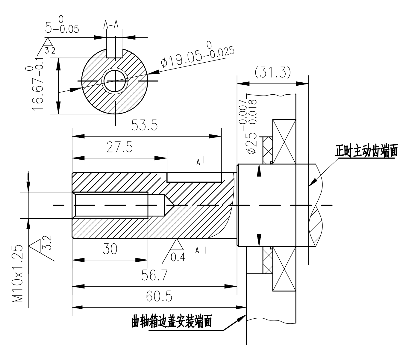
曲轴输出端简图
