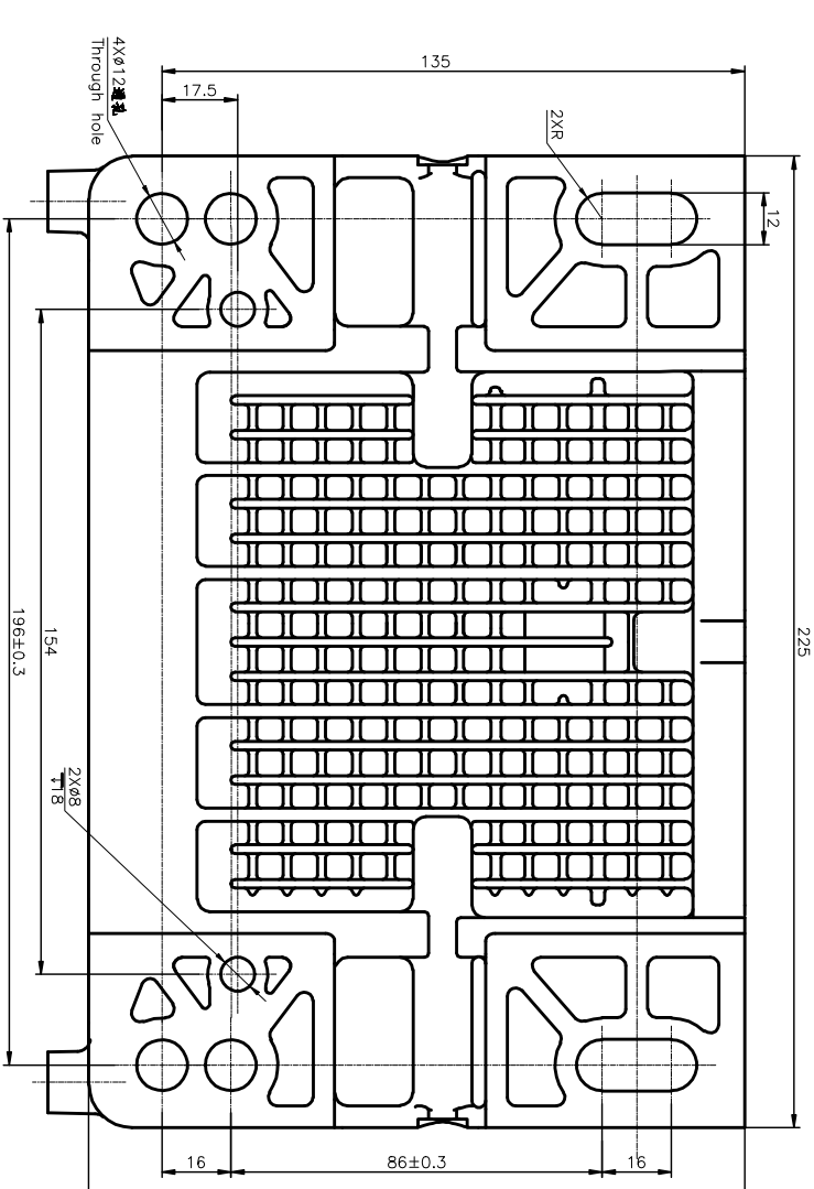
底座安裝尺寸
