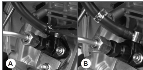
Рис. 9 Хомут топливного шланга
