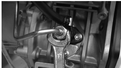
Рис. 12 Удаление воздуха из топливного насоса
