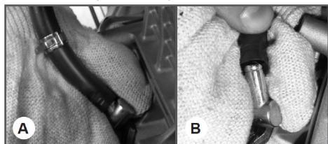
Рис. 10 Снятие топливного шланга
