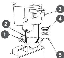
Рис. 23 Обслуживание фильтра-отстойника
