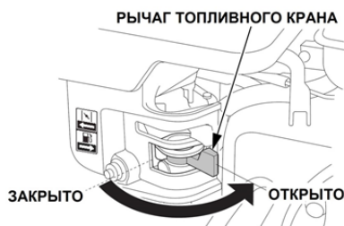
Рис. 14 Рычаг топливного крана
