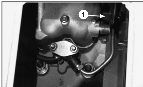
Рис. 13 Рычаг декомпрессора
