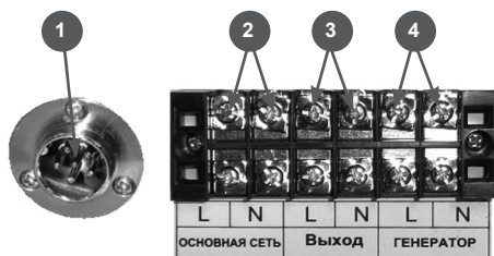
Рис. 15 Панель подключения блока ATS
