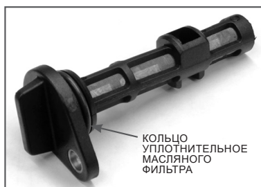
Рис. 19 Масляный фильтр
