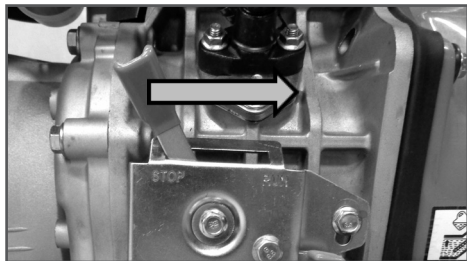
Рис. 11 Рычаг включения ТНВД
