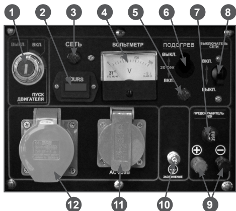
Рис. 3 Панель управления
