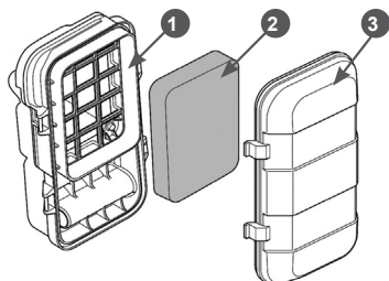
Рис. 14 Обслуживание воздушного фильтра
