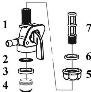
Рис. 16 Устройство топливного крана
