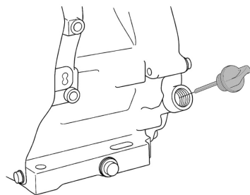
Рис. 6 Крышка-щуп маслозаливной горловины
