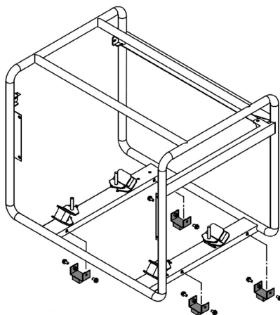
Рис. 4 Установка опор рамы
