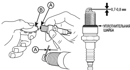
Рис. 19 Проверка зазора между электродами
