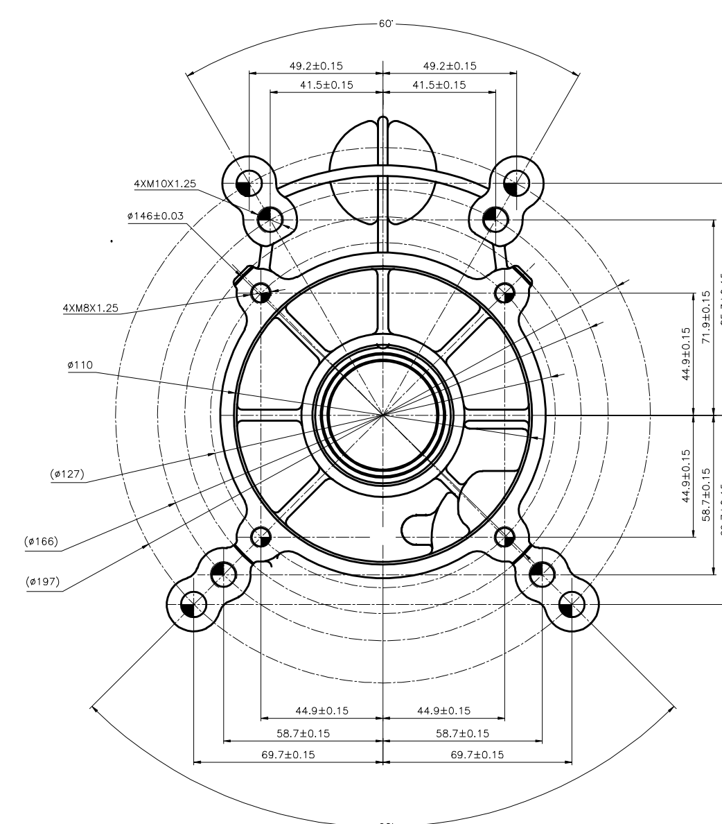
箱盖接口尺寸
