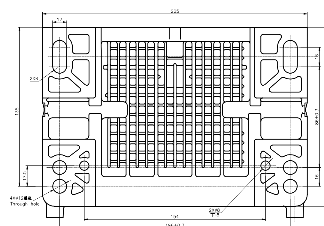
底座安裝尺寸
