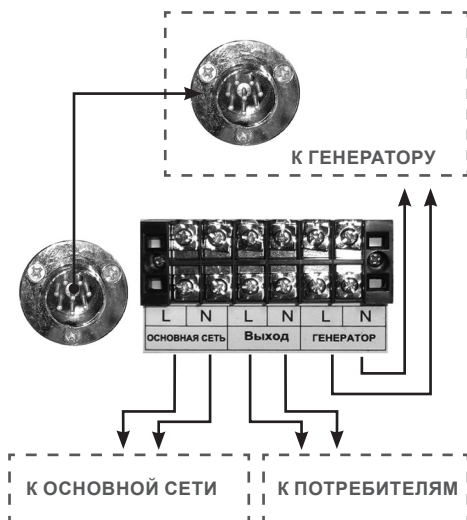
Рис. 16 Схема подключения блока ATS
