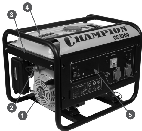
Рис. 1 Общий вид
