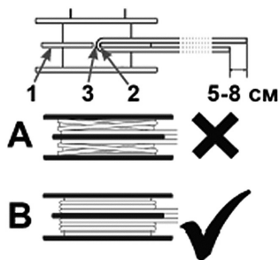
Рис. 10 Намотка корда
