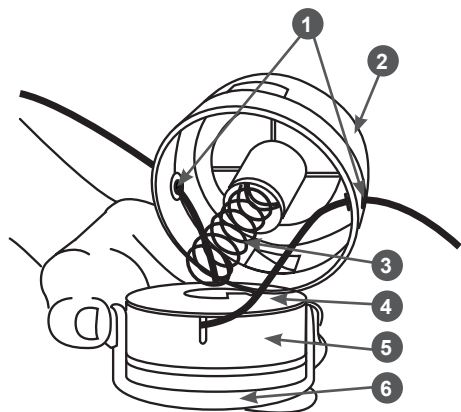
Рис. 9 Снятие катушки
