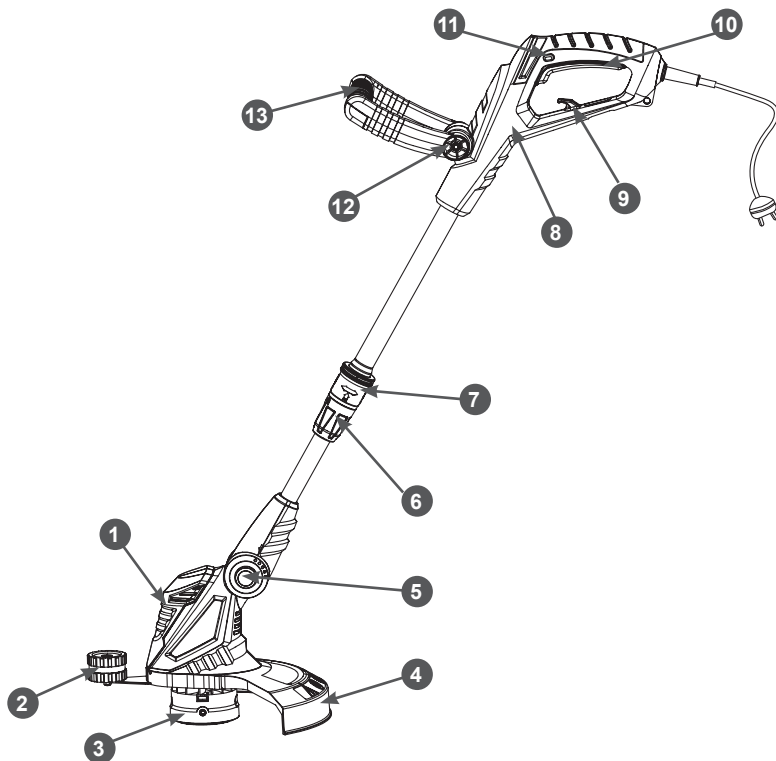
Рис. 1 Основные узлы и органы управления
