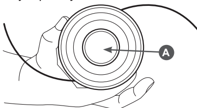
Рис. 8 Снятие крышки триммерной головки
