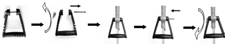
Рис. 3 Установка передней рукоятки
