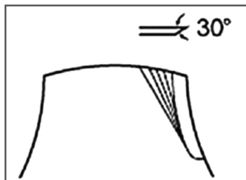
Рис. 20 Заточка ножа
