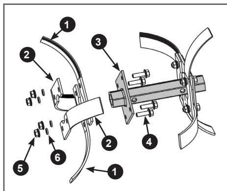
Рис. 16 Установка ножей на внутренний фланец основной секции оси фрезы
