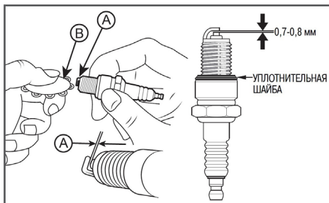
Рис. 38 Проверка межэлектродного зазора
