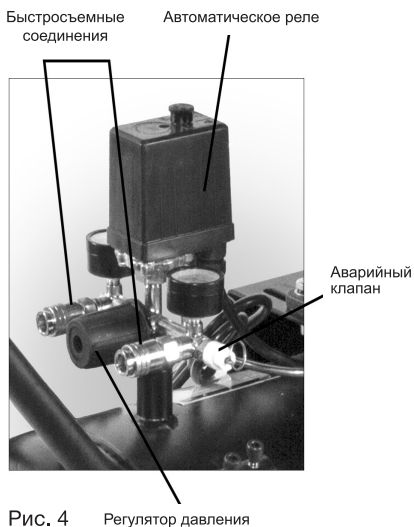
Рис. 4 Регулятор давления
