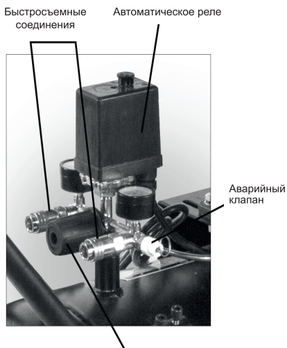
Рис. 4 Регулятор давления
