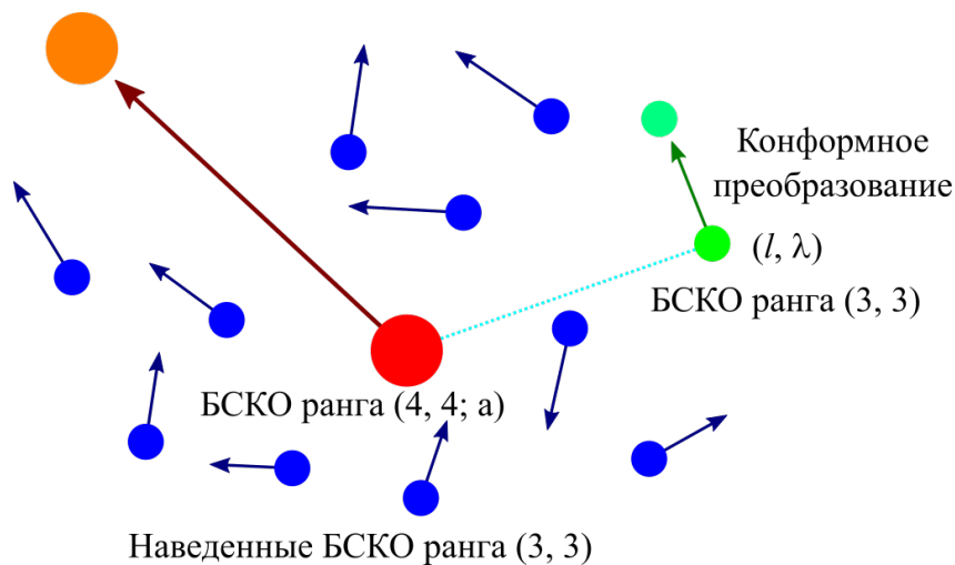
Рис. 4. Конформное преобразование одной из наведённых БСКО ранга (3, 3), соответствующей опорным элементам l и \lambda , вызывает неконформное смещение исходной БСКО ранга (4, 4; а). Это, в свою очередь, приводит к неконформному смещению всех остальных наведённых БСКО ранга (3, 3)
