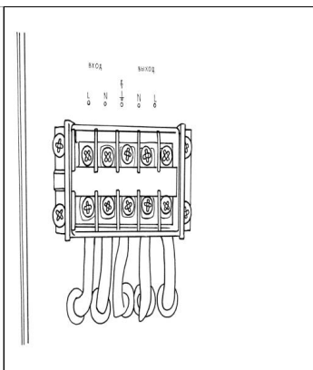
Рис. 6. Схема подключения
