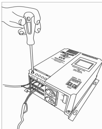
Рис 7. Подключение стабилизатора
