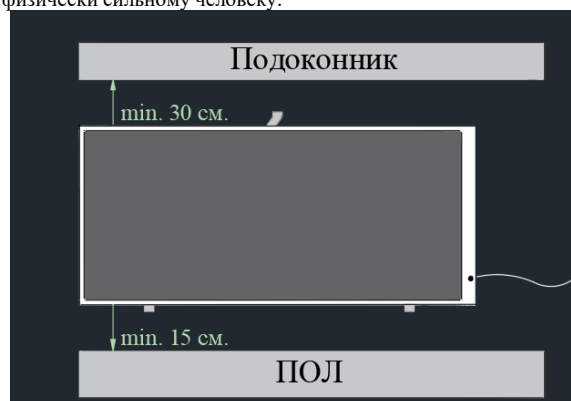
Рис.1 Крепление обогревателя к стене под подоконником.
