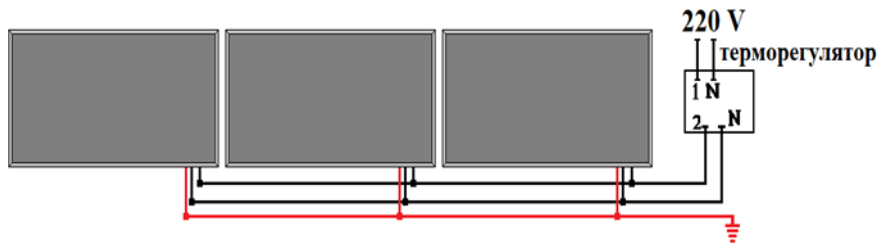
Рисунок 2. Подключение обогревателей к терморегулятору.
