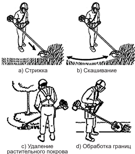
Рис. 11 Движение триммера
