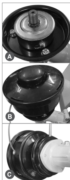
Рис. 6 Установка триммерной головк
